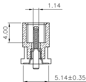
剖面 A-A 比例 1: 1
